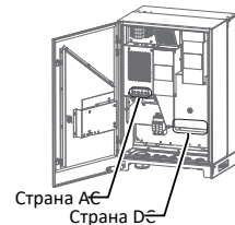
Fig. 7: Присъединителни клеми
