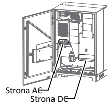
Rys. 7: Zaciski przyłączeniowe
