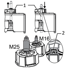
SI 14: Podloga opiaščanja na privitju EMV
