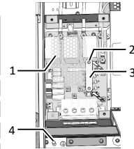
Fig. 3: 5-проводниково свързване
