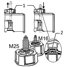
Fig. 14: Apantallamiento en el racor EMV
