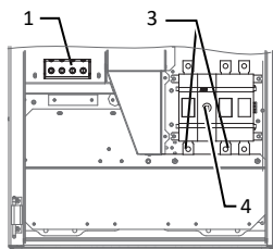
Obr. 4: Připojovací svorky - verze Basic Obr. 5: Připojovací svorky verze M
