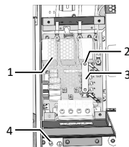
Fig. 3: 5-leders-tilkobling
