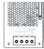
Fig. 8: 4-ledaranslutning
