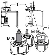
איור 14: מגן בחיבור הברגה EMC
