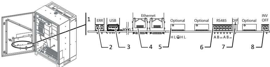
Fig. 13: Πλακέτα επικοινωνίας: Σύνδεση και αντιστοίχιση των θυρών
