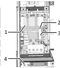
Abb. 3: 5-Leiter Anschluss
