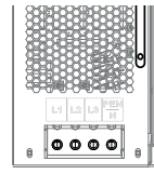
Obr. 8: 4vodičové připojení
