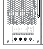
Kuva 8: 4-johdinliitännä
