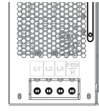
Fig. 8: 4-ledertilslutning
