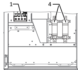
Rys. 6: Zaciski przyłączeniowe: Wersja S
