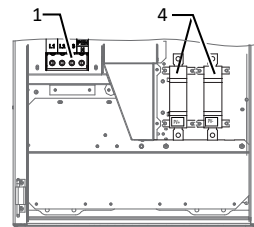
Fig. 6: Присъединителни клеми: Версия S
