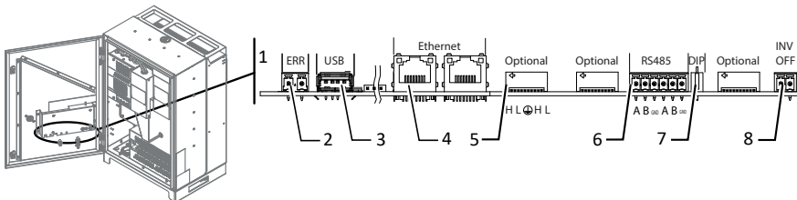
Fig. 13: Kommunikasjonkort: Tilkobling og tildeling av grensesnittene
