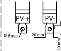
Fig. 10: Tilslutning til S-variant
