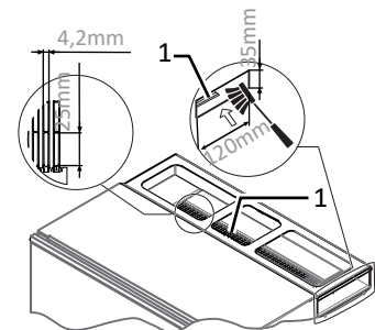
Abb. 69: Kühlrippen reinigen
