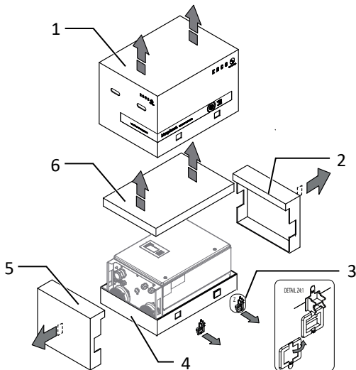
Abb. 11: Kartonage öffnen
