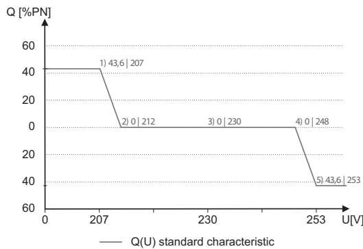
Abb. 51: Q(U) Standard Kennlinie mit 5 Stützstellen
