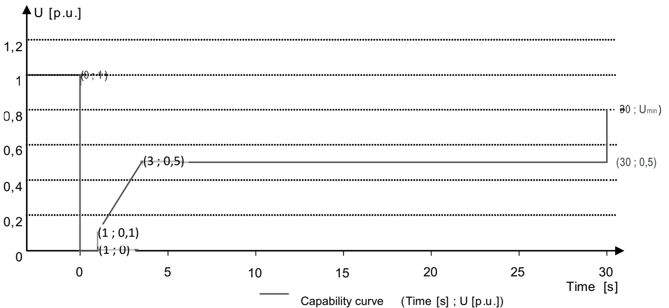
Abb. 60: Störfestigkeitskennlinie bezogen auf die Nennspannung (p.u.) des blueplanet 125.0TL3
