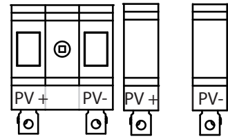
Abb. 76: DC Leitungen trennen
