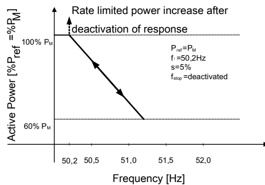
Abb. 59: Beispielverhalten ohne Hysterese (Modus 2)
