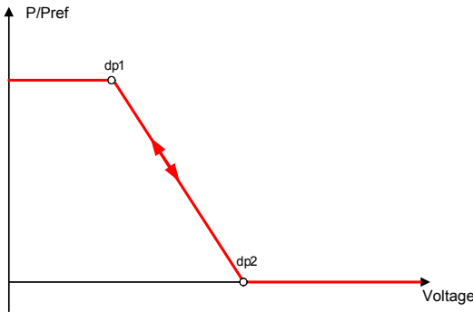
Abb. 52: Beispiel-Kennlinie ohne Hysterese
