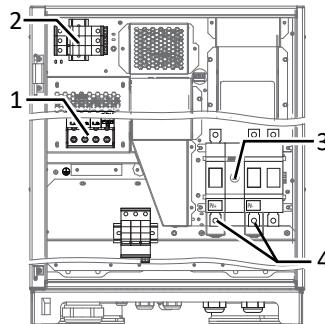
Abb. 23: Anschlussklemmen M-Version
