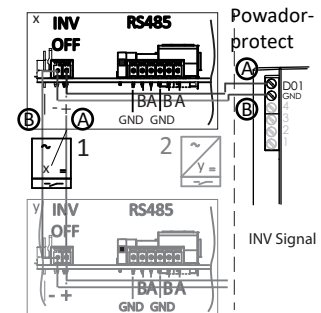
Abb. 44: Gerät mit Powador-protect verbinden
