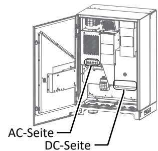
Abb. 25: Anschlussklemmen
