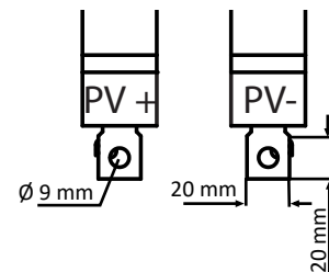
Abb. 35: Anschluss an S-Variante
