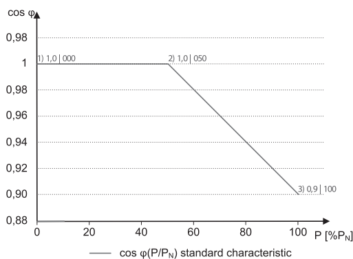
Abb. 50: cos φ / (P/Pn) Standard Kennlinie mit 3 Stützstellen
