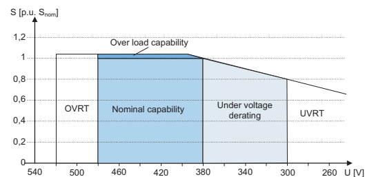
Abb. 49: Scheinleistungabhängigkeit der Netzspannung
