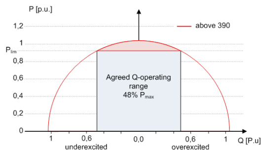
Abb. 65: P-Q-Betriebsbereich mit begrenzter Wirkleistung ( Q_{max} = S_{max} \neq P_{max} ) für PV-Wechselrichter
