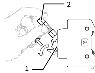
Abb. 72: DC-Sicherung einlegen
