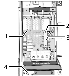
Abb. 21: 5-Leiter Anschluss
