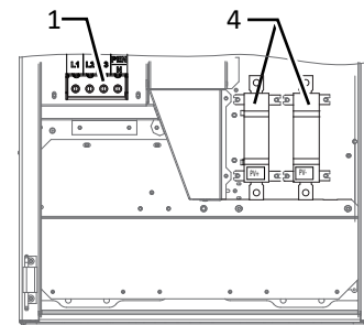
Abb. 24: Anschlussklemmen: S-Version
