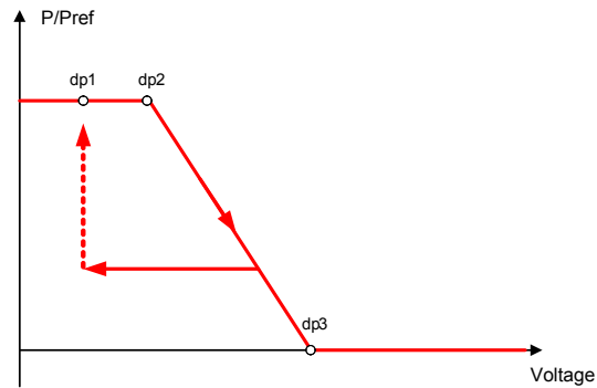
Abb. 53: Beispiel-Kennlinie mit Hysterese und einer Deaktivierungsschwelle unterhalb der Aktivierungsschwelle
