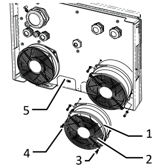
Abb. 70: Lüfter demontieren
