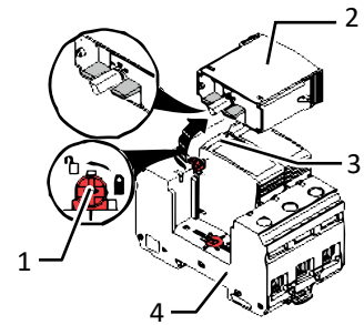
Abb. 74: DC-Ueberspannungsschutz
