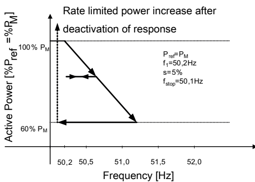
Abb. 58: Beispielverhalten mit Hysterese (Modus 1)
