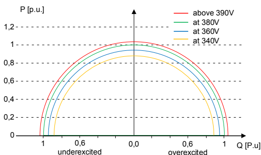
Abb. 48: P-Q Betriebsbereich für blueplanet 50.0TL3
