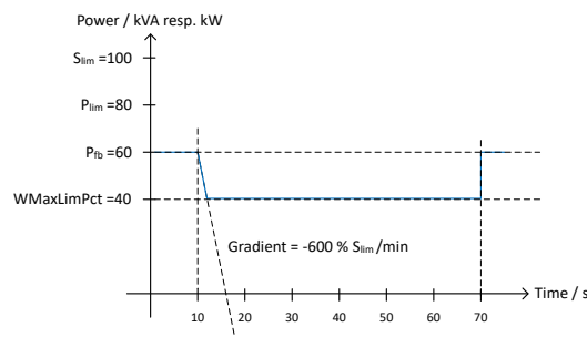
Abb. 66: Leistungsgradient gemäß Musterparameter und Berechnung
