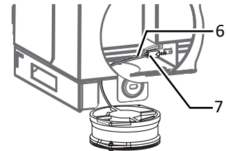
Abb. 71: Lüfterstecker abziehen
