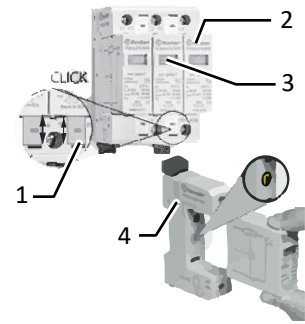
Abb. 73: AC-Ueberspannungsschutz
