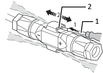
Abb. 75: Steckverbinder abstecken
