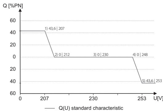
Abb. 40: Q(U) Standard Kennlinie mit 5 Stützstellen
