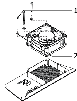
Abb. 60: Austauschlüfter einbauen
