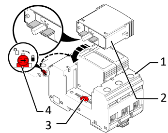
Abb. 25: DC-Überspannungsschutz einsetzen
