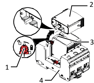
Abb. 61: DC-Überspannungsschutz
