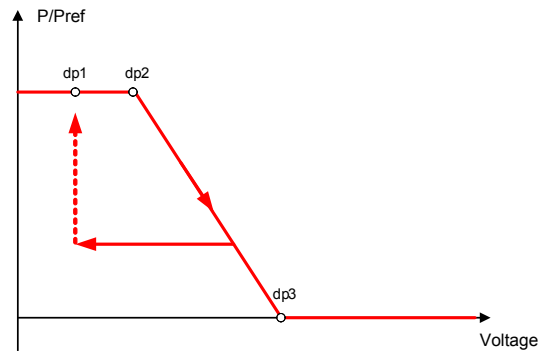
Abb. 42: Beispiel-Kennlinie mit Hysterese und einer Deaktivierungsschwelle unterhalb der Aktivierungsschwelle
