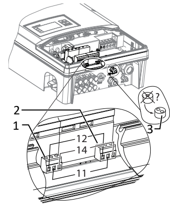
Abb. 26: Überspannungsschutz mit Fernmeldeüberwachung verbinden
