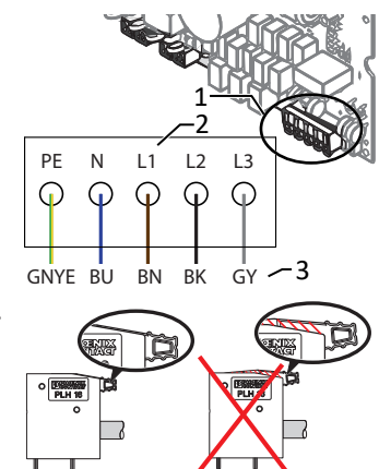
Abb. 17: AC-Anschlussklemme 5-polig
