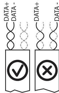
Abb. 31: Belegung der verdrehten Adernpaare
