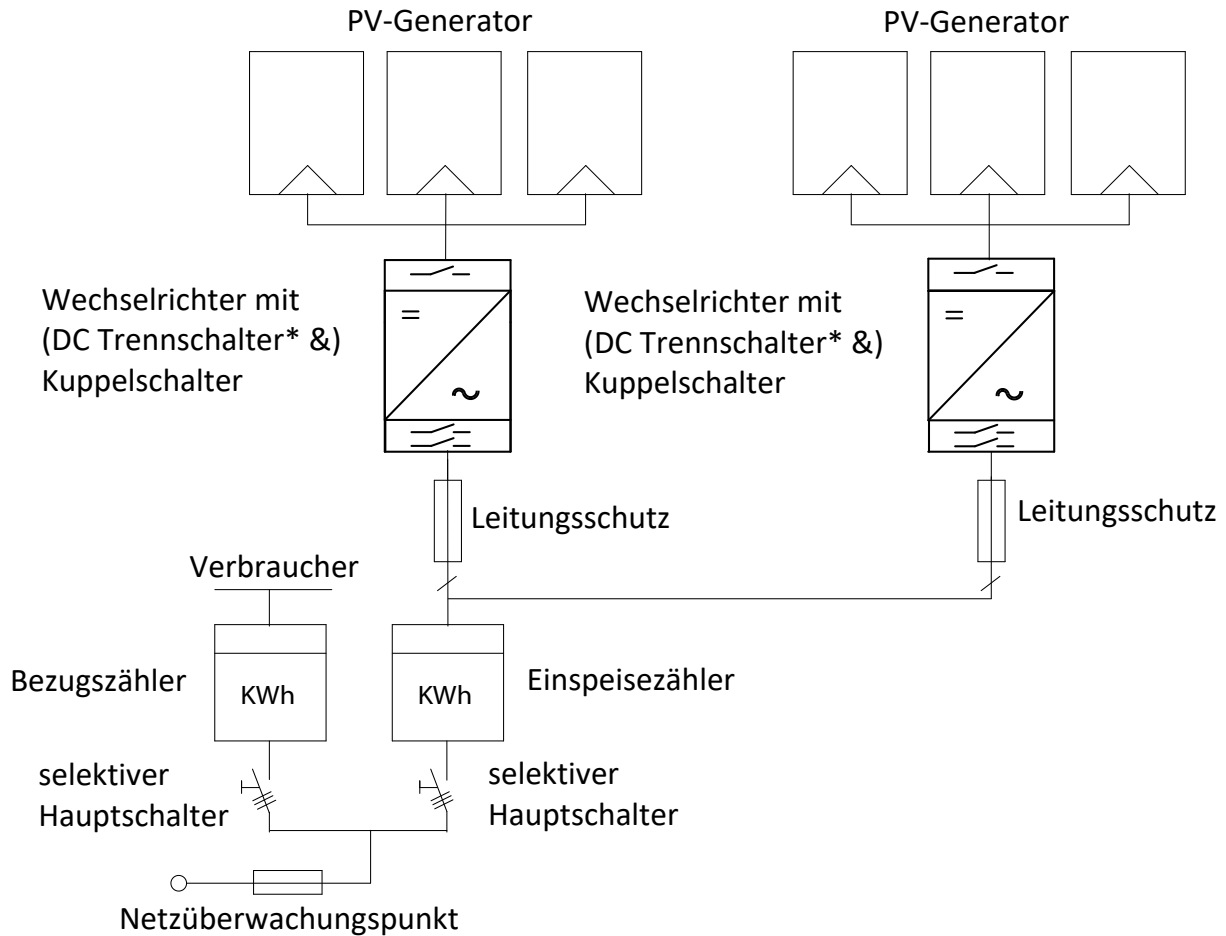
Abb. 5: Übersichtsschaltplan für eine Anlage mit zwei Wechselrichtern
