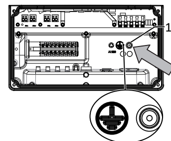
Abb. 27: Erdungspunkt
