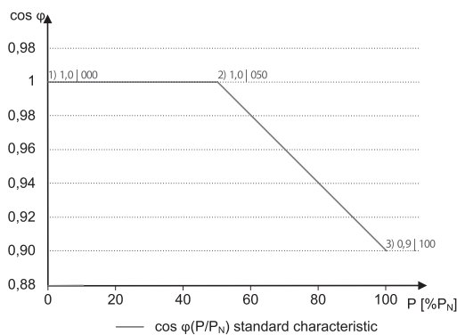
Abb. 39: \cos \varphi / (P/P_n) Standard Kennlinie mit 3 Stützstellen
