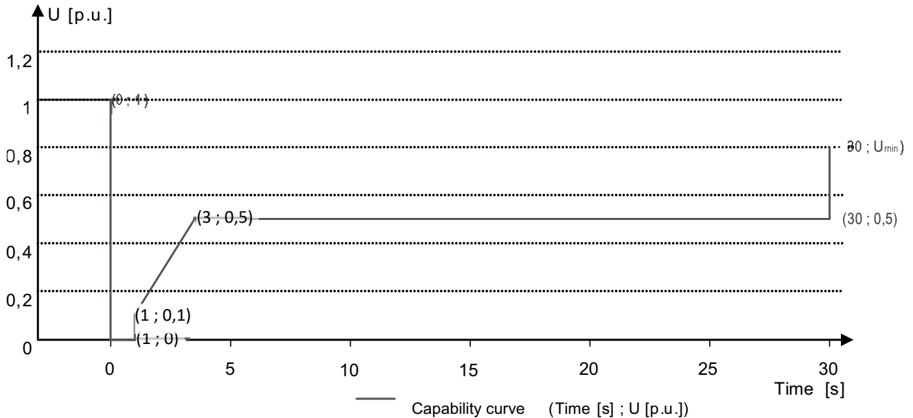
Abb. 49: Störfestigkeitskennlinie bezogen auf die Nennspannung (p.u.) des blueplanet 125.0TL3
