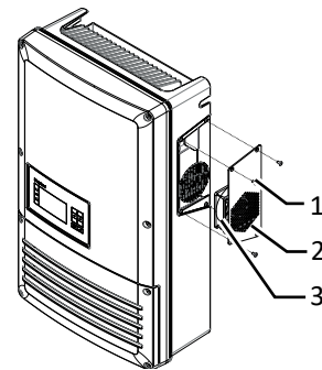
Abb. 59: Abdeckung mit Lüfter demonstrieren
