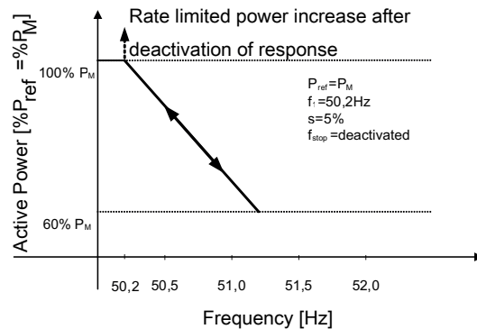
Abb. 48: Beispielverhalten ohne Hysterese (Modus 2)
