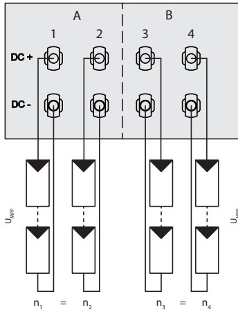
Abb. 18: Empfohlene Standardbeschtaltung
