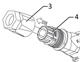
Abb. 22: Einsatz in Hülse schieben
