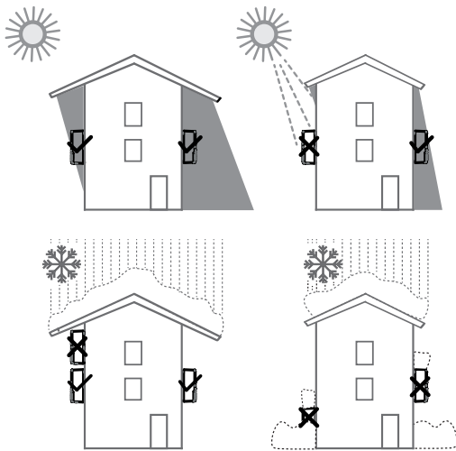
Abb. 8: Gerät bei Außeninstallation
