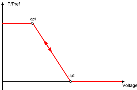
Abb. 41: Beispiel-Kennlinie ohne Hysterese
