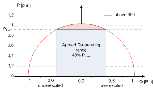
Abb. 54: P-Q-Betriebsbereich mit begrenzter Wirkleistung ( Q_{max}=S_{max} \neq P_{max} ) für PV-Wechselrichter
