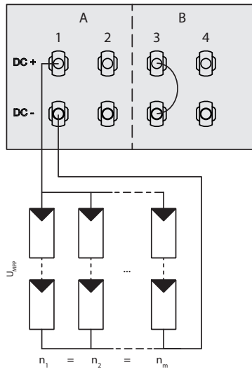
Abb. 19: Parallele Eingangsbeschtaltung mit Y-Adapter, Kurzschluss des nicht verwendeten MPP-Trackers B
