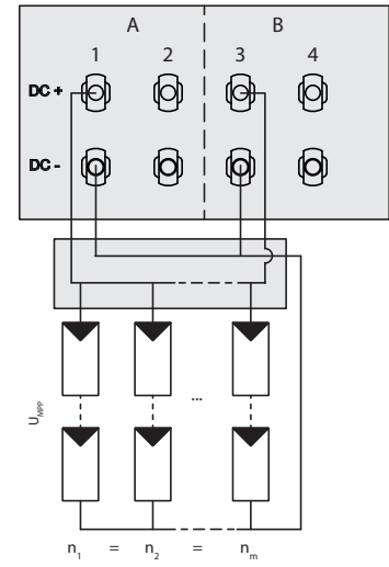
Abb. 20: Ein Generator parallel auf beiden MPP-Trackern
