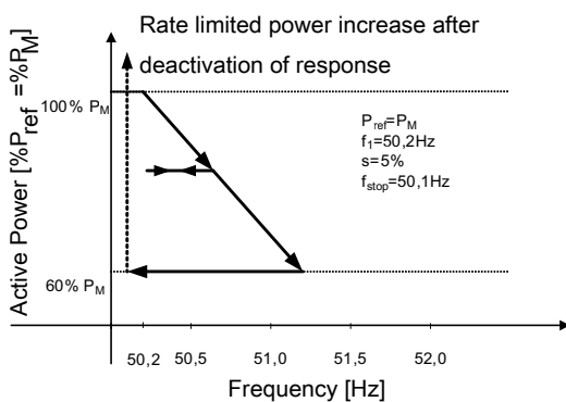
Abb. 47: Beispielverhalten mit Hysterese (Modus 1)
