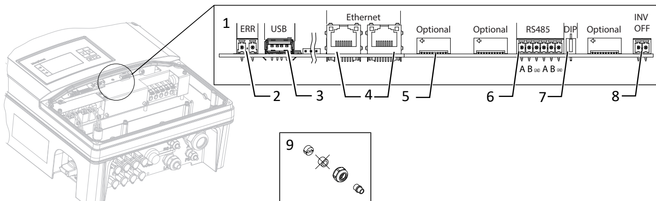
Abb. 28: Kommunikationsplatine (HMI-Platine)
