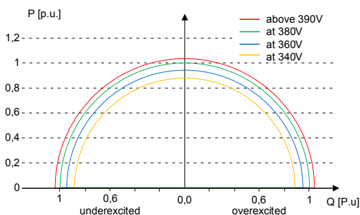
Abb. 37: P-Q Betriebsbereich für Geräte über 12 kVA
