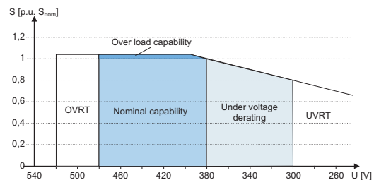
Abb. 38: Scheinleistung abhängig der Netzspannung
