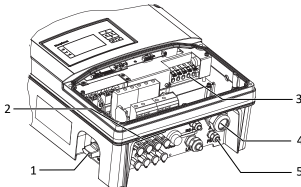
Abb. 16: Anschlussbereich
