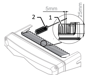
Abb. 58: Kühlrippen reinigen
