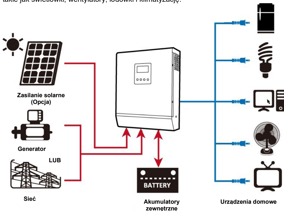
Rysunek 1 Hybrydowy układ zasilania
